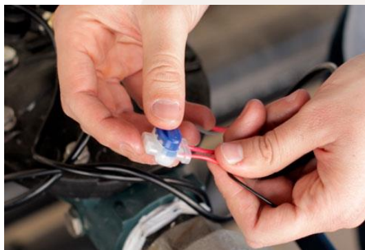
Figura 6. Conexión de la polaridad positiva mediante un conector estanco.
